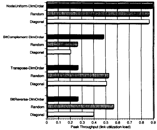
(b) 16 x 16 torus
