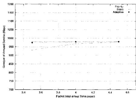
Fig. 8. Goodput of AF service
